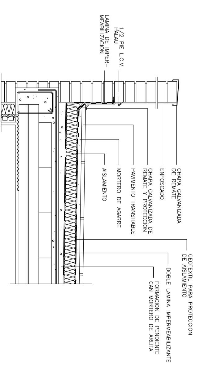
REFORMA CUBIERTA PLANA TRANSITABLE NORMAL
